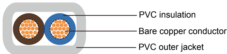
H03V2V2H2-F
