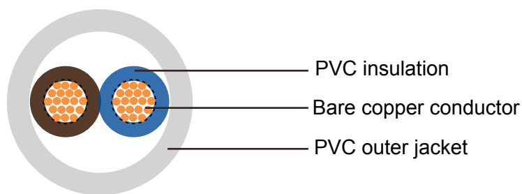
H03VV-F
